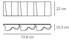
Logico parete mini 3 in linea HALO max 3x52W (E 27) – ES
