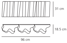
Logico parete 3 in linea HALO max 6x52W (E 27) – ES
