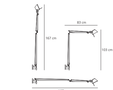
Tolomeo braccio HALO max 1x70W (E27) - ES IP20
