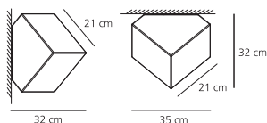
Edge parete/soffitto 21 FLUO 1x20W (E 27) – TC-TSE
