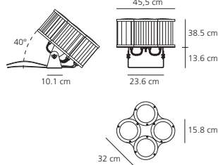
Metaponto HALO 3x150W (B 15d) – ES
