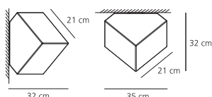
Edge parete/soffitto 30 FLUO 1x23W (E 27) – TC-TSE
