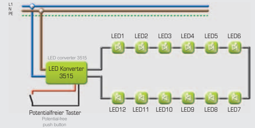
Reihenschaltung, max. Leitungslänge sekundärseitig 10m series connexion, max. length of connection cable secondary side 10m
