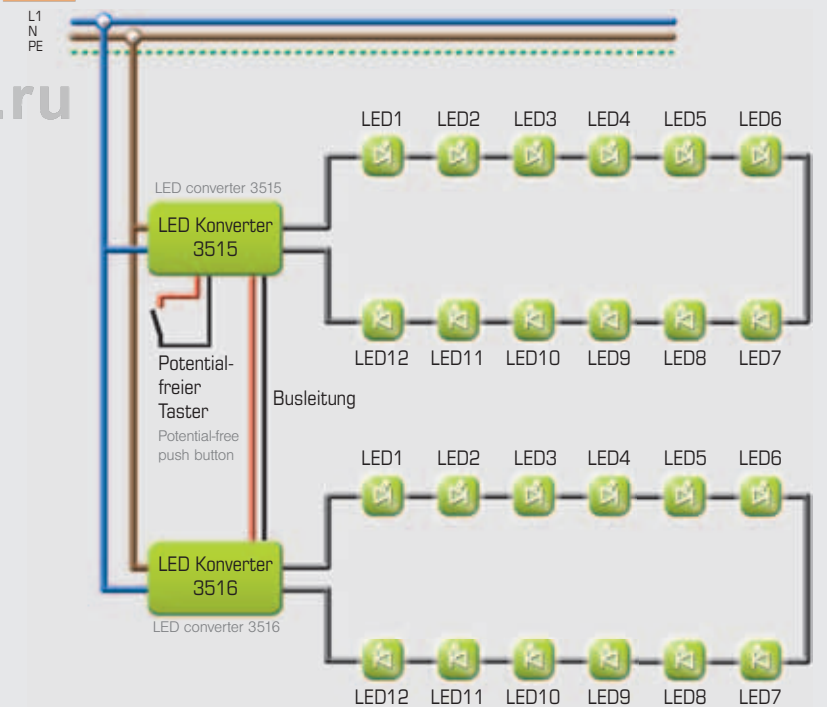
Reihenschaltung, max. Leitungslänge sekundärseitig 10m series connexion, max. length of connection cable secondary side 10m
