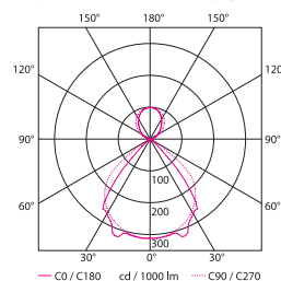
d-LEATHER 1xT16 54W
