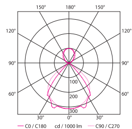
d-BEEF 1xT16 54W
