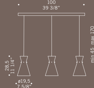
MEMORY S3GL 3x70W E27 alogeno chiara clear halogen 3x75W E27-PAR 30 3x20W E27 fluorescente fluorescent
