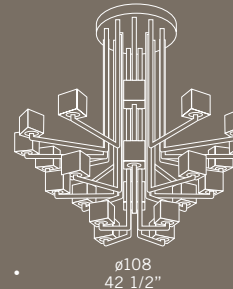
OTTO X OTTO K4+8+12 24x60W G9 alogeno bispina halogen bi-pin doppia accensione double switch
