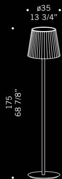
LUMÈ R1 1x60W E27 Globolux chiara clear Globolux 1x70W E27 alogeno chiara clear halogen con variatore with dimmer
