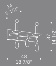
ELORO A2 2x40W E14 sferetta chiara little sphere
