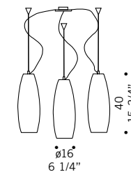
PERONI S16D3 3x70W E27 alogeno chiara clear halogen 3x75W E27 - PAR 30 3x23W E27 fluorescente fluorescent cavo elettrico 200 cm cables lenght 200 cm
