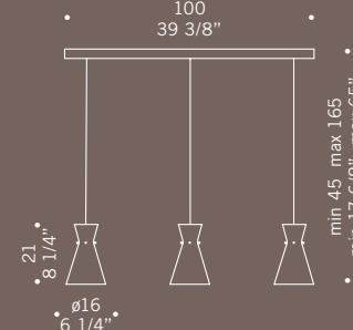
MEMORY S3PL 3x70W E27 alogeno chiara clear halogen 3x75W E27-PAR 30
