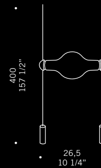
ADAM CV 120W R7s alogena lineare 114 mm halogen linear 114 mm con varia luce potenza max totale 500W dimmer total power max 500W
