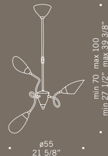
POLI PÒ K3 3x40W E14 sferetta chiara little sphere
