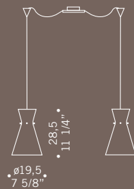
MEMORY S2GD 2x70W E27 alogeno chiara clear halogen 2x75W E27-PAR 30 2x20W E27 fluorescente fluorescent cavo elettrico 200 cm cables lenght 200 cm
