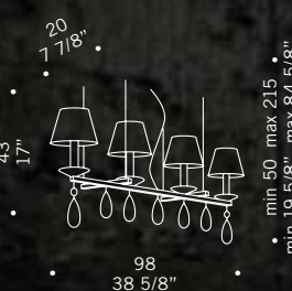
ELORO S4L SHADE 4x40W E14 sferetta chiara little sphere
