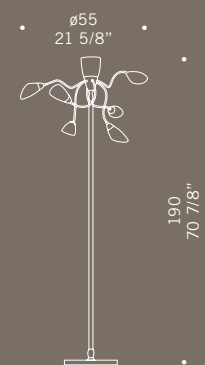
POLI PÒ R 6x40W E14+ sferetta chiara little sphere 1x150W E27 alogeno chiara clear halogen con variatore with dimmer
