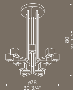
OTTO X OTTO K4+8 12x60W G9 alogeno bispina halogen bi-pin doppia accensione double switch
