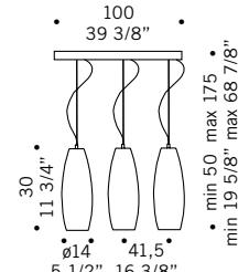
PERONI S14L 3x70W E27 alogeno chiara clear halogen 3x50W E27 - PAR 20 3x23W E27 fluorescente fluorescent
