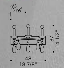
NOTO A3 3x40W E14 sferetta chiara little sphere
