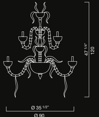
L 1052 6+3 x 40 W E14 max
