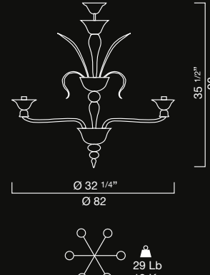
L 1008/NZ 6 x 40 W E14 max
