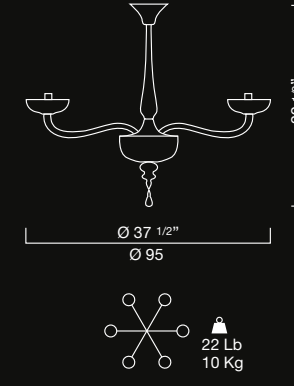
L 1006 6 x 40 W E14 max
