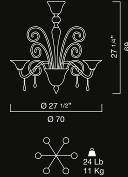
L 1014/6 6 x 40 W E14 max
