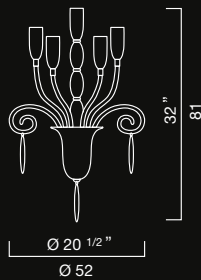
L 1027/APPLIQUE 5 x 40 W E14 max
