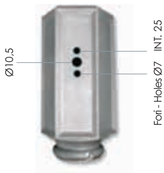
ART. 6081-A-2 2 luci - 2 lights
