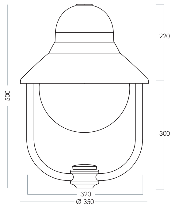
Con art. 5904-A-2 - With art. 5904-A-2
