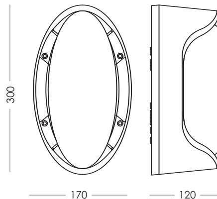
Esempio senza art. 4102-A Example without art. 4102-A
