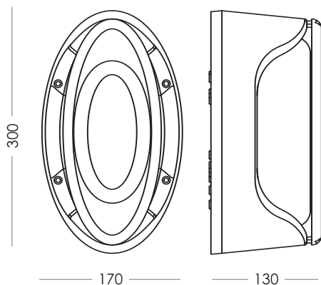
Esempio con art. 4102-A Example with art. 4102-A
