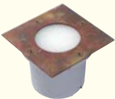
247.08.A0 L 13x13cm ↓10cm 1x Max 6W Gx53 MICROLINX IP 65 ▲
