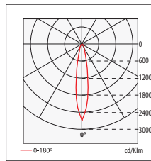
n° 91 HIT-T 150W-10° BUBO PR-0913 \eta=70.5\%
