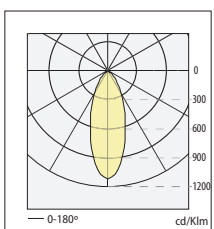
n° 29 TRIMIUM E HIT-T 150W 40° η=70.600 %
