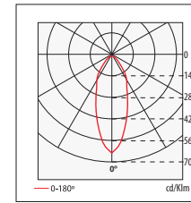
n° 92 HIT-T 150W-45° BUBO PR-0914 \eta=68.4\%
