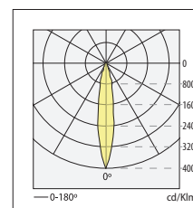
n° 28 TRIMIUM E HIT-T 150W 12° η=80.100 %
