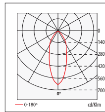
n° 90 HIT-T 70W-45° BUBO PR-0912 \eta=68.4\%
