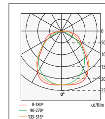
n° 95 TL5 G5-3x24W BORBOLETA \eta=61,52\%
