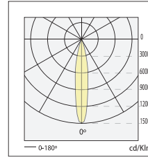
n° 19 CDM-R111 70W 24° η=100 %
