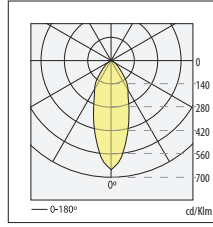
n° 82 MACH1 HIT-T 70W 45° \eta=50.500\%
