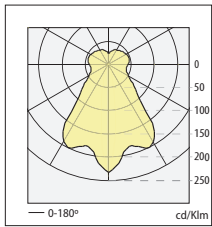
n° 84 FILIPA HIT-T 70W con reflector B9 \eta=73.400\%
