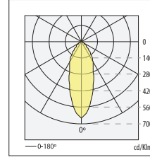
n° 22 MACH1 HIT-T 150W 45° η=50.500 %
