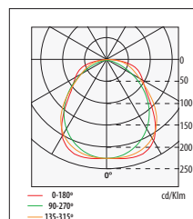
n° 93 TL5 G5-3x14W BORBOLETA AD-0616 \eta=61,52\%
