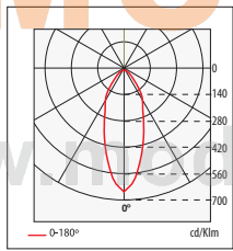
n° 88 HIT-T 35W-45° BUBO PR-0910 \eta=68.4\%
