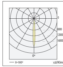
n° 18 CDM-R111 70W 10° η=100 %
