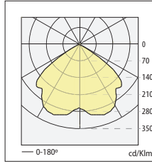
n° 27 TRIMIUM 2x18W η=66.600 %
