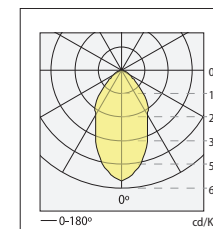
n° 31 TRIMIUM S130 QT-TC 60W η=64.900 %
