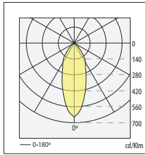
n° 81 MACH1 HIT-T 35W 45° \eta=50.500\%
