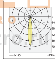
n° 25 DUPLO 8x PowerLed 1W η=87.54 %
