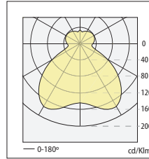
n° 85 FILIPA G PL-H 120W con reflector B9 \eta=78.600\%
