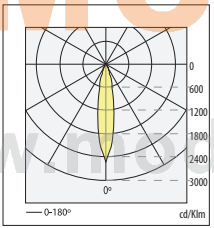
n° 24 DUPLO QT-TC 60W η=60.200 %
