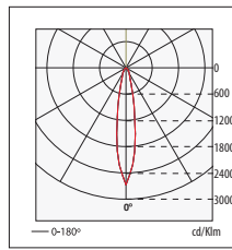
n° 87 HIT-T 35W-10° BUBO PR-0909 \eta=70.5\%
