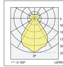
n° 83 FILIPA P QT-TC 60W \eta=70\%
