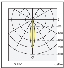
n° 23 DUPLO HIT-TC 70W η=60.200 %
