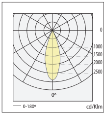
n° 20 CDM-R111 70W 40° η=100 %
