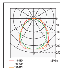
n° 94 TL5 G5-2x14W BORBOLETA \eta=61,52\%
