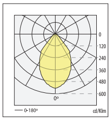
n° 26 TRIMIUM HIT-DE 70W η=65.600 %
