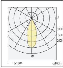
n° 17 CDM-R111 35W 40° η=100 %
