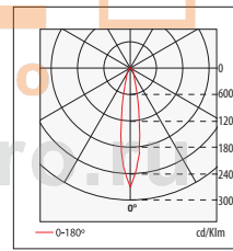
n° 89 HIT-T 70W-10° BUBO PR-0911 \eta=68.4\%
