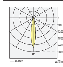
n° 21 MACH1 HIT-T 70W 10° η=56.000 %
