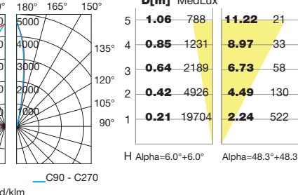
Reflector A
