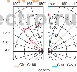
Reflector B
