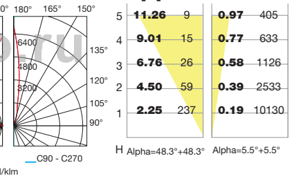
Reflector A
