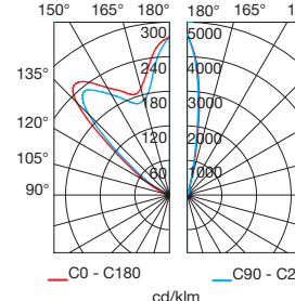
Reflector B
