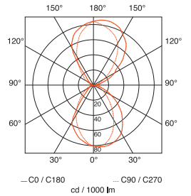
PL 23W
