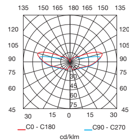
PL 13W
