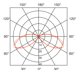
PL 23W
